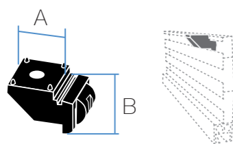
AA206 Clip a soffitto
